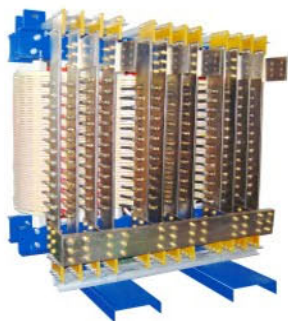
干式电炉变压器
